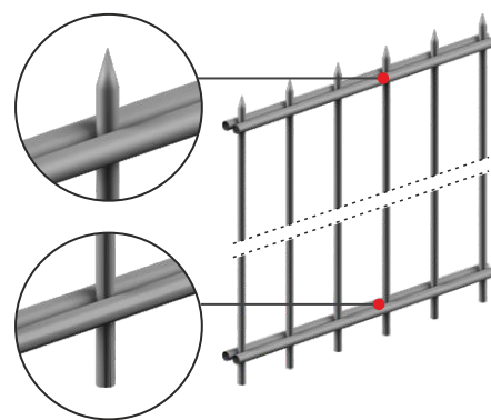
EINSEITIG ANGESPITZT
