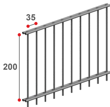
MW 35 x 200
