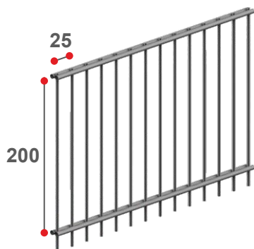
MW 25 x 200
